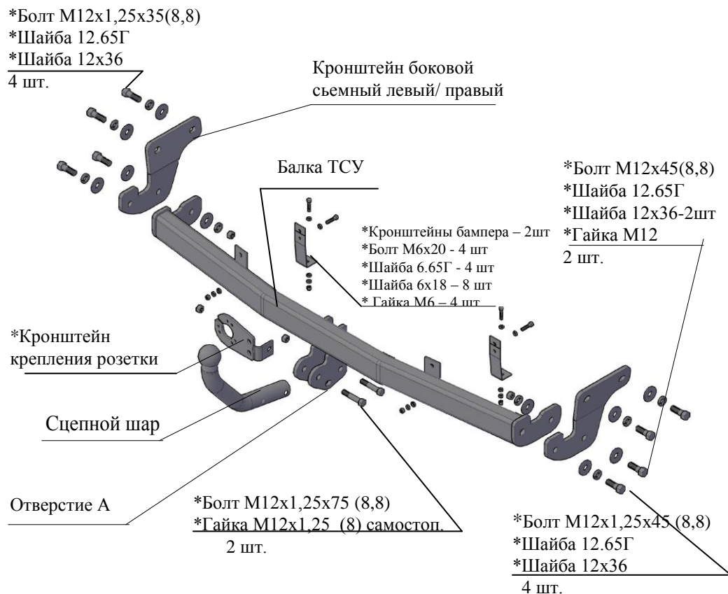
Рис.1 Тягово-сцепное устройство ТСУ 7241.
