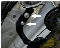
Рис. 2 - Установка заднего кронштейна
