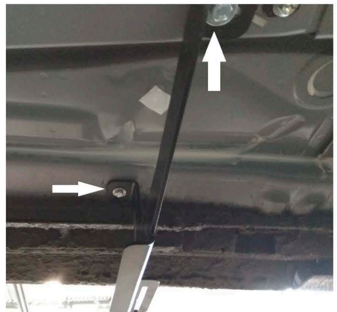
Рис. 4 - Установка переднего кронштейна
